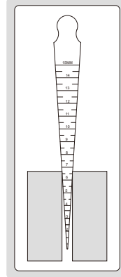
楔形塞尺测量缝隙宽度
